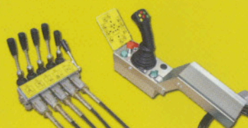
Comandi a cavo flessibili Cable controls Commande à câbles Fernbedienung mit 4 Bowdenzüge
